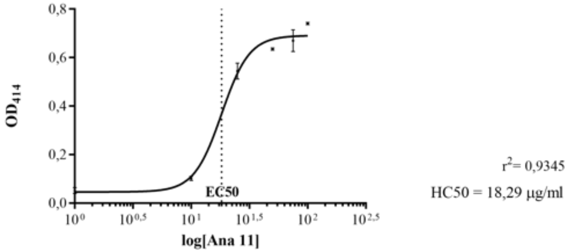
Şekil 4.64. Ana 11 peptidinin hemolitik aktivitesini gösteren HC 50 grafiği.
