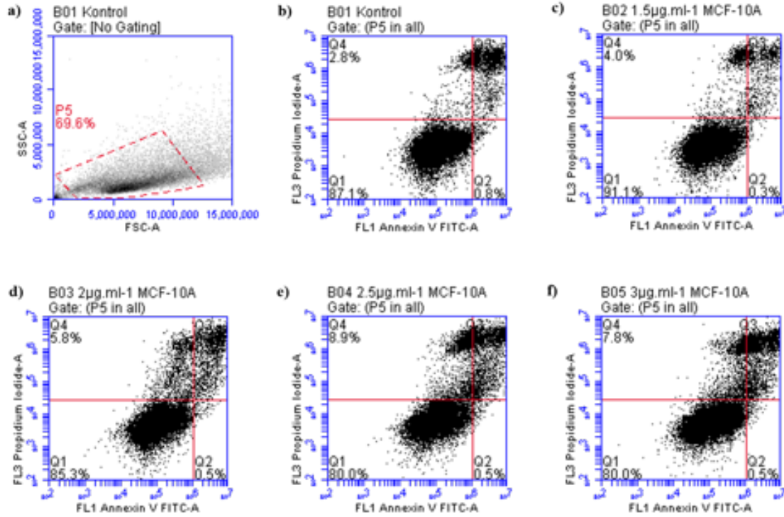
Şekil 4.80. MCF-10A hücre hattının akış sitometrisi ile gerçekleştirilen apoptoz analizi grafikleri. a) Uygulama verilmeyen kontrol grubuna ait ışık saçılım grafiği ve debris dışındaki hücre grubunu temsil eden P5 kapısı, b) kontrol, c) 1,5 µg/ml, d) 2 µg/ml, e) 2,5 µg/ml ve f) 3 µg/ml Ana 11 uygulanan hücrelerin AV/FITC – PI floresan yoğunluğu grafikleri. Kadranın etrafındaki alanlardan Q1: canlı, Q2: erken apoptotik, Q3: geç apoptotik, Q4: nekrotik hücreleri temsil etmektedir.
