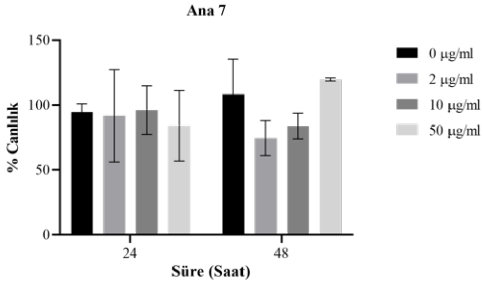
Şekil 4.24. Ana 7 fraksiyonunun her bir dozunun 24 ve 48 saat sonunda MDA-MB-231 hücre hattı üzerindeki % canlılık etkisini gösteren bar grafiği.
