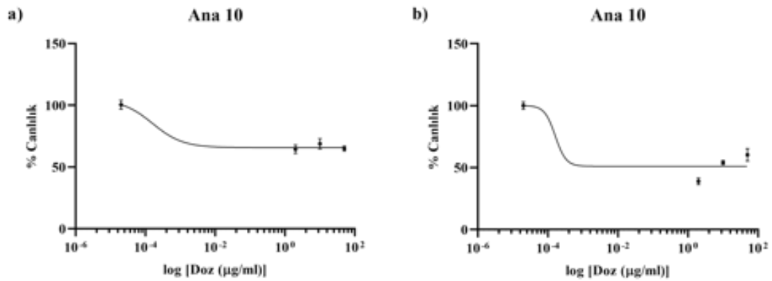
Şekil 4.37. Ana 10 fraksiyonunun MCF-7 hücre hattı üzerindeki sitotoksik etkisi. Ana 10 fraksiyon dozuna bağlı olarak a) 24 saat, b) 48 saat sonundaki cevabı gösteren eğriler.
