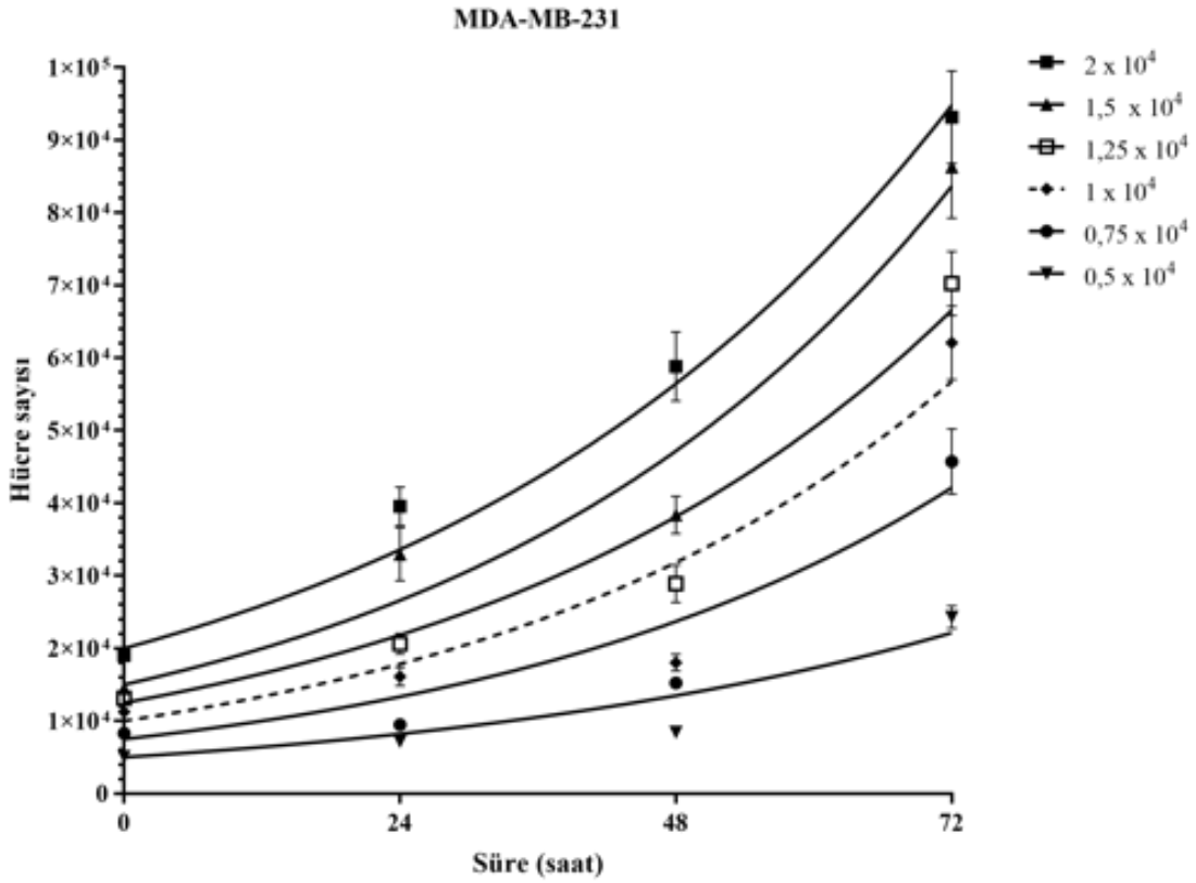
Şekil 4.9. MDA-MB-231 hücre hattına ait büyüme eğrisi grafiği.
