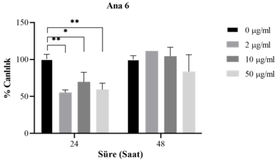
Şekil 4.22. Ana 6 fraksiyonunun her bir dozunun 24 ve 48 saat sonunda MCF-7 hücre hattı üzerindeki % canlılık etkisini gösteren bar grafiği.
