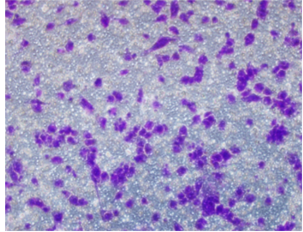
Şekil 4.67. Transwell invazyon testi için MDA-MB-231 hücre hattı kullanılarak gerçekleştirilen optimum hücre sayısı denemesinin 10X ve 40X büyütme ile inverted mikroskop altında görüntülenmesiyle elde edilen fotoğraflar.
