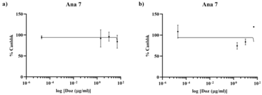
Şekil 4.23. Ana 7 fraksiyonunun MDA-MB-231 hücre hattı üzerindeki sitotoksik etkisi. Ana 7 fraksiyon dozuna bağlı olarak a) 24 saat, b) 48 saat sonundaki cevabı gösteren eğriler.
