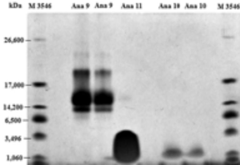
Şekil 4.8. Majör fraksiyon Ana 9, 10 ve 11'in denatüre edici Tricine-SDS PAGE görüntüleri. Her bir kuyuya 15 µg fraksiyon yüklenmiştir.
