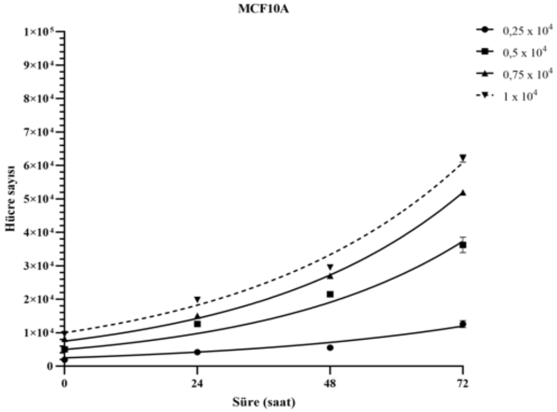
Şekil 4.11. MCF-10A hücre hattına ait büyüme eğrisi grafiği.
