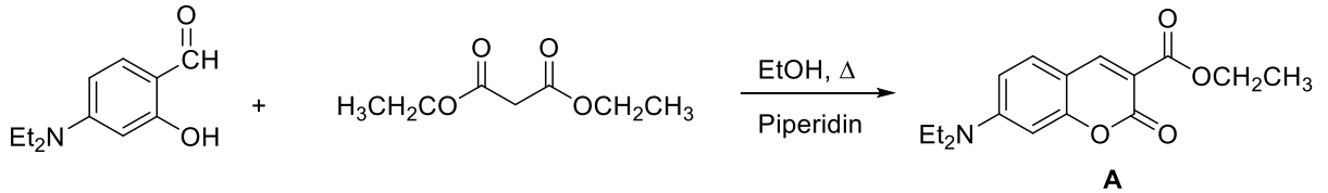
Şekil 4.1. Etil 7-(dietilamino)-2-okso-2 H -kromen-3-karboksilat (A) bileşiğinin sentez şeması.
