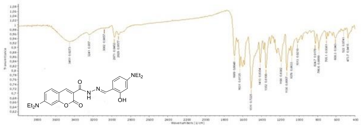
A6. 2 Nolu Bileşiğin FT-IR (KBr) Spektrumu
