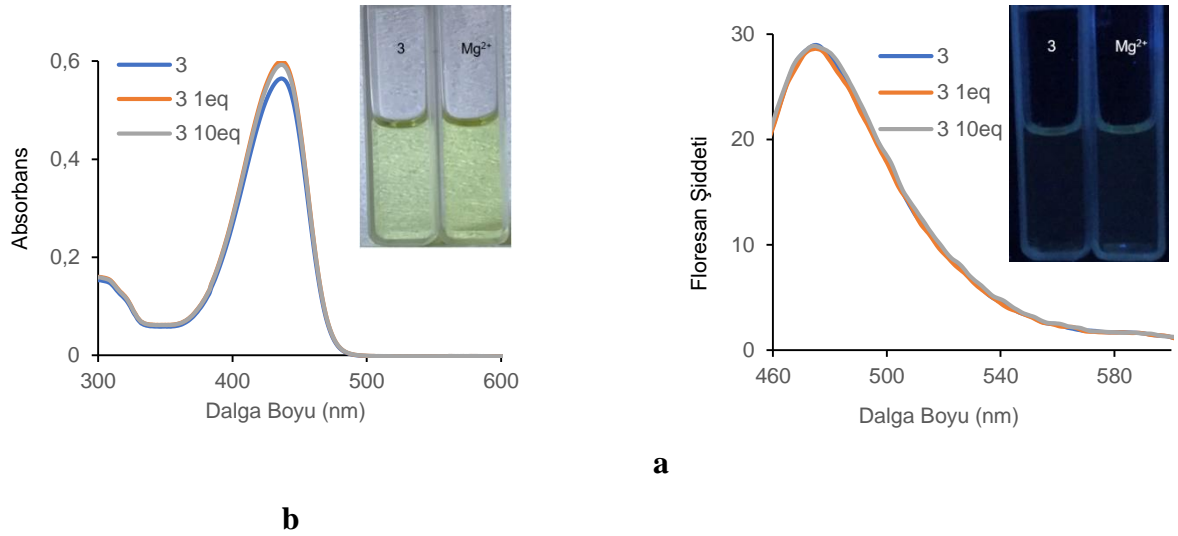
Şekil 5.60. 3 nolu bileşiğin MgCl 2 ile titrasyonu sonucu elde edilen absorpsiyon ( 1 \times 10^{-5} M DMSO çözücüsünde) (a) ve emisyon ( 1 \times 10^{-6} M DMSO çözücüsünde, \lambda_{ex} = 440 nm) (b) spektrumları. (Grafiklerin içerisinde 3 nolu bileşiğin MgCl 2 ile titrasyonu sonucu gözlenen fotofiziksel değişiklikler gün ışığında (a) ve UV ışığında (365 nm) (b) gözlenen fotoğrafları)
