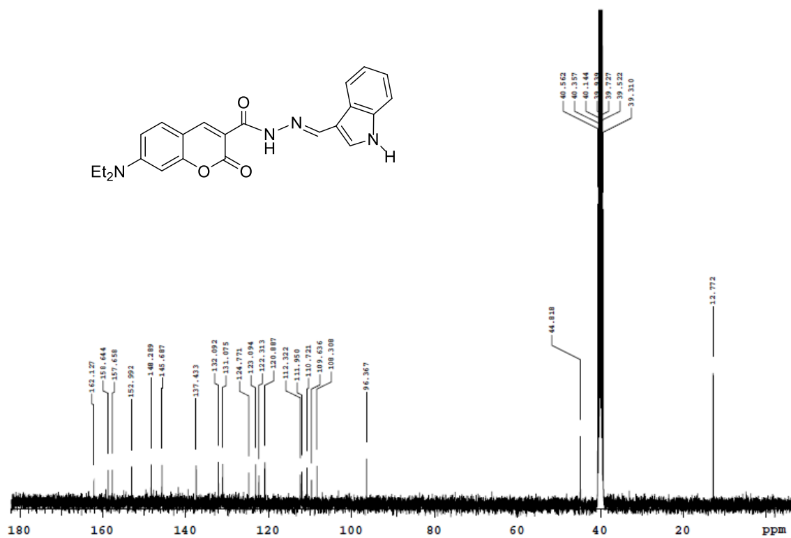
A12. 3 Nolu Bileşğin 13 C-NMR Spektrumu DMSO d 6 Çözücüsünde
