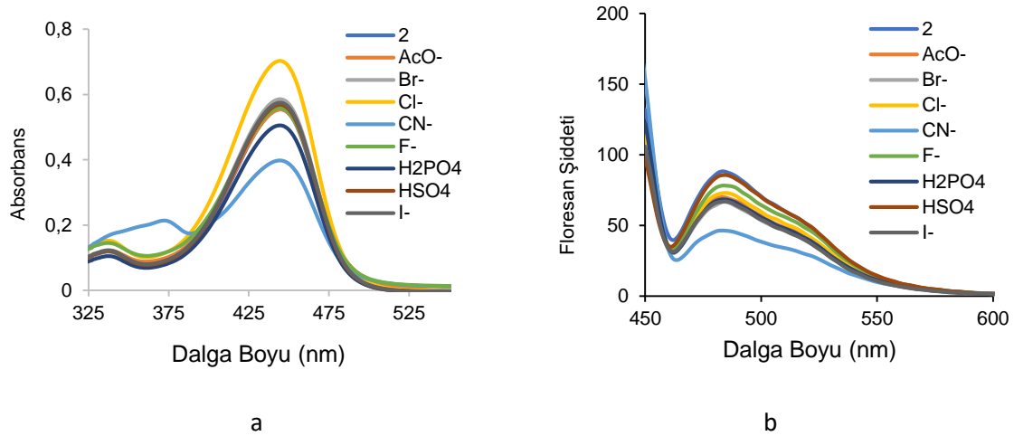
Şekil 5.25. 2 nolu bileşimin çeşitli tetrabütülamonyum tuzlarının 20 eşdeğer mol eklenmesi sonucu elde edilen absorpsiyon ( 1 \times 10^{-5} \text{M} DMSO çözücüsünde) (a) ve emisyon ( 1 \times 10^{-6} \text{M} DMSO çözücüsünde) (b) spektrumları
