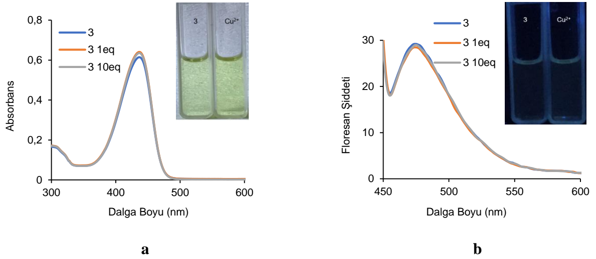
Şekil 5.59. 3 nolu bileşiğin CuCl 2 ile titrasyonu sonucu elde edilen absorpsiyon ( 1 \times 10^{-5} M DMSO çözücüsünde) (a) ve emisyon ( 1 \times 10^{-6} M DMSO çözücüsünde, \lambda_{ex} = 440 nm) (b) spektrumları. (Grafiklerin içerisinde 3 nolu bileşiğin CuCl 2 ile titrasyonu sonucu gözlenen fotofiziksel değişiklikler gün ışığında (a) ve UV ışığında (365 nm) (b) gözlenen fotoğrafları)
