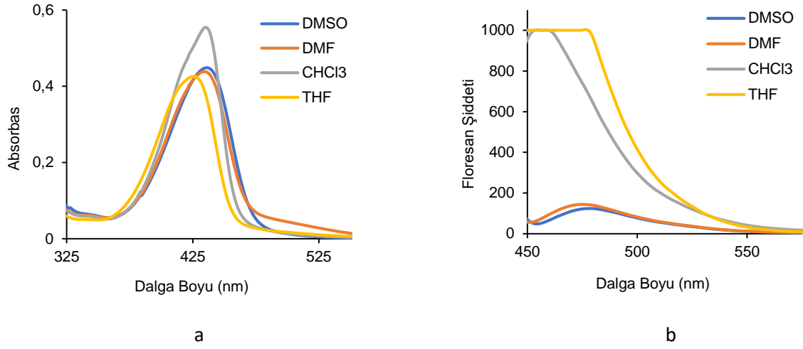
Şekil 5.63. 4 nolu bileşiğinin farklı çözücüler içerisindeki Absorpsiyon (a) ( 1 \times 10^{-5} M DMSO çözücüsünde) ve Emisyon (b) Spektrumları ( 1 \times 10^{-6} M DMSO çözücüsünde)
