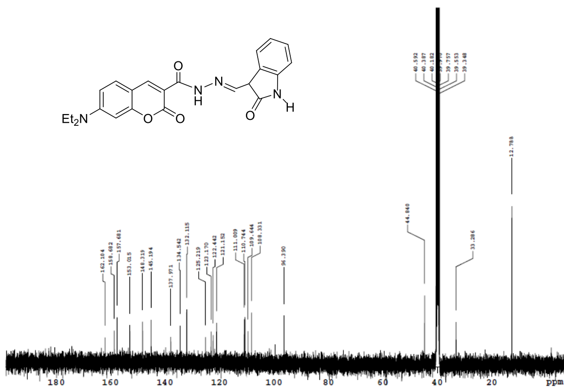
A20. 5 Nolu Bileşğin 13 C-NMR Spektrumu DMSO d 6 Çözücüsünde
