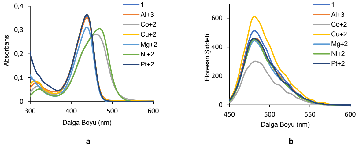
Şekil 5.15. 1 nolu bileşiğine çeşitli katyon klorür tuzlarının 20 eşdeğer mol eklenmesi sonucu elde edilen absorpsiyon ( 1 \times 10^{-5} M DMSO çözücüsünde) (a) ve emisyon ( 1 \times 10^{-6} M DMSO çözücüsünde, \lambda_{ex} = 438 nm) (b) spektrumları
