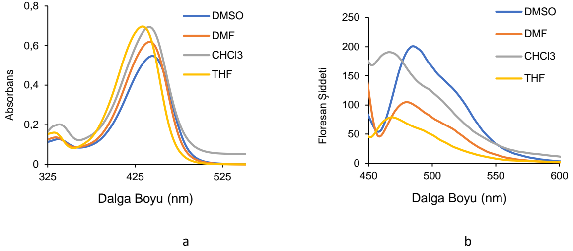
Şekil 5.23. 2 nolu bileşğin farklı çözücüler içerisindeki Absorpsiyon (a) ( 1 \times 10^{-5} M DMSO çözücüsünde) ve Emisyon (b) Spektrumları ( 1 \times 10^{-6} M DMSO çözücüsünde)
