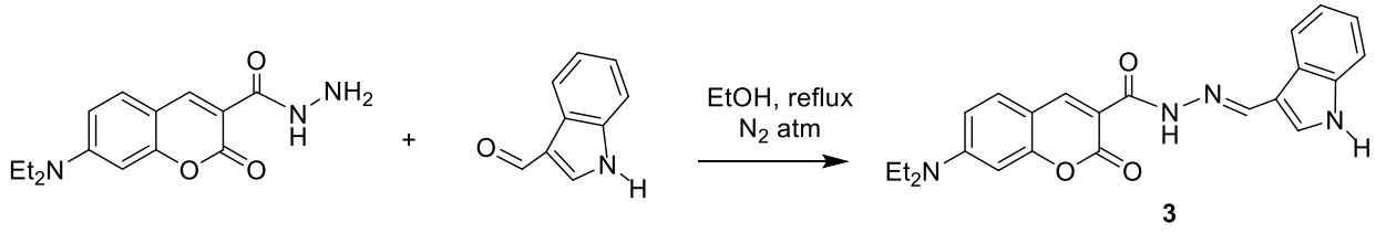
Şekil 4.5. (E)-N'-((1H-indol-3-il) metilen)-7-(dietilamino)-2-okso-2H-kromen-3-karbohidrazid (3) bileşiğinin sentez şeması.
