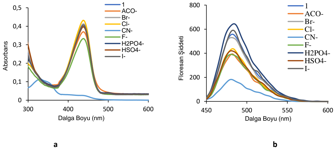
Şekil. 5.5. 1 nolu bileşiğine çeşitli tetrabutilamonyum tuzlarının 20 eşdeğer mol eklenmesi sonucu elde edilen absorpsiyon ( 1 \times 10^{-5} \text{M} DMSO çözücüsünde) (a) ve emisyon ( 1 \times 10^{-6} \text{M} DMSO çözücüsünde, \lambda_{\text{ex}} = 440 \text{ nm} ) (b) spektrumları
