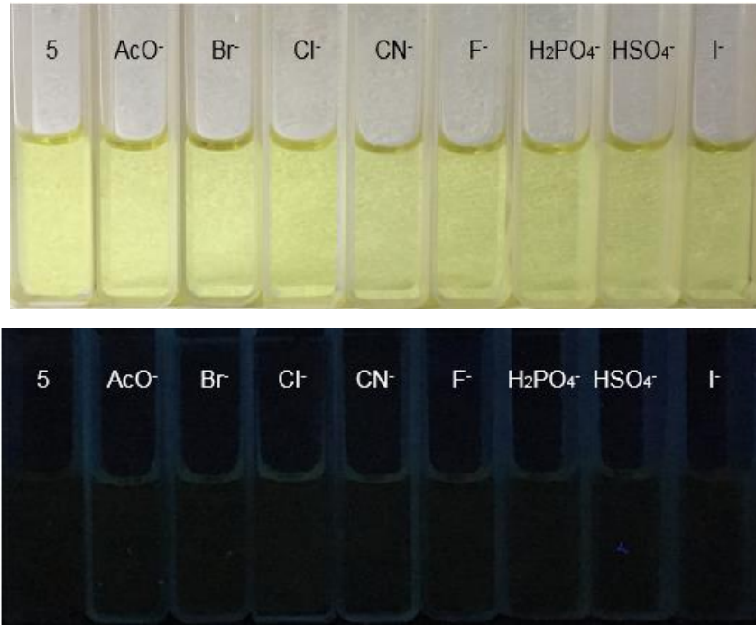
Şekil 5.86. 5 nolu bileşiğine tetrabutülamonyum tuzlarının eklenmesi sonucu gözlenen fotofiziksel değişiklikler gün ışığında (üst) ve UV ışığında (365 nm) (alt) gözlenen fotoğrafları
