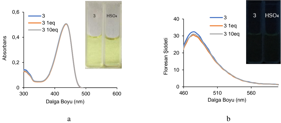
Şekil 5.53. 3 nolu bileşiğin TBAHSO 4 ile titrasyonu sonucu elde edilen absorpsiyon ( 1 \times 10^{-5} M DMSO çözücüsünde) (a) ve emisyon ( 1 \times 10^{-6} M DMSO çözücüsünde, \lambda_{ex} = 440 nm) (b) spektrumları. (Grafiklerin içerisinde 3 nolu bileşiğin TBAHSO 4 ile titrasyonu sonucu gözlenen fotofiziksel değişiklikler gün ışığında (a) ve UV ışığında (365 nm) (b) gözlenen fotoğrafları)
