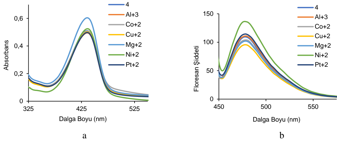
Şekil 5.75. 4 nolu bileşiğine çeşitli katyon klorür tuzlarının 20 eşdeğer mol eklenmesi sonucu elde edilen absorpsiyon ( 1 \times 10^{-5} M DMSO çözücüsünde) (a) ve emisyon ( 1 \times 10^{-6} M DMSO çözücüsünde, \lambda_{ex} = 440 nm ) (b) spektrumları
