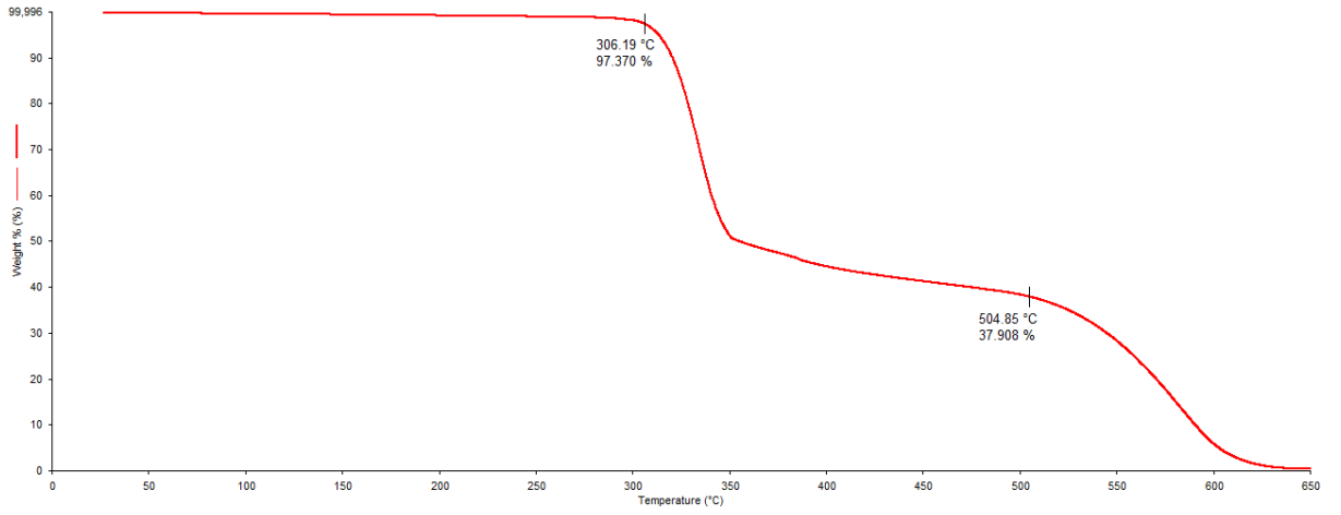
Şekil 5.105. 3 Nolu Bileşiğin Termogravimetrik Bozunma Grafiği
