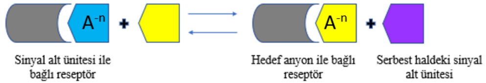
Şekil 2.3. Bir yer değiştirme yaklaşımına dayalı anyon sensör sistem
