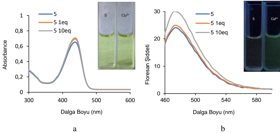
Şekil 5.99. 5 nolu bileşiğin \text{CuCl}_2 ile titrasyonu sonucu elde edilen absorpsiyon ( 1 \times 10^{-5} M DMSO çözücüsünde) (a) ve emisyon ( 1 \times 10^{-6} M DMSO çözücüsünde, \lambda_{\text{ex}} = 440 nm) (b) spektrumlar. (Grafiklerin içerisinde 5 nolu bileşiğin \text{CuCl}_2 ile titrasyonu sonucu gözlenen fotofiziksel değişiklikler gün ışığında (a) ve UV ışığında (365 nm) (b) gözlenen fotoğrafları)
