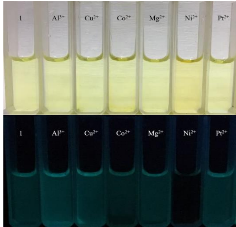
Şekil 5.16. 1 nolu bileşiğine çeşitli katyon klorür tuzlarının eklenmesi sonucu gözlenen fotofiziksel değişiklikler gün ışığında (üst) ve UV ışığında (365 nm) (alt) gözlenen fotoğrafları
