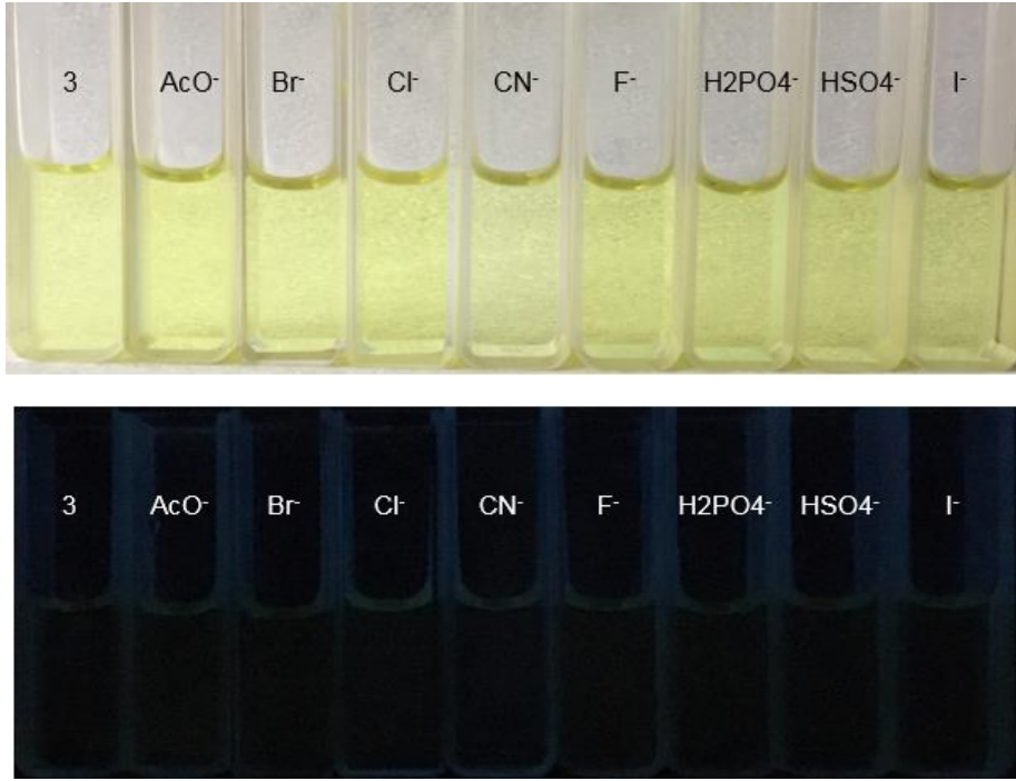
Şekil 5.46. 3 nolu bileşiğine tetrabutilamonyum tuzlarının eklenmesi sonucu gözlenen fotofiziksel değişiklikler gün ışığında (üst) ve UV ışığında (365 nm) (alt) gözlenen fotoğrafları
