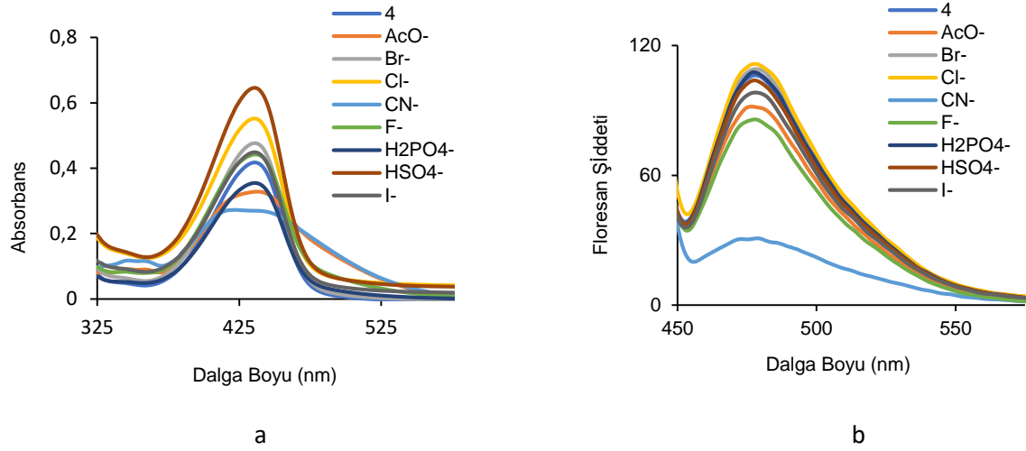
Şekil 5.65. 4 nolu bileşiğine çeşitli tetrabutülamonyum tuzlarının 20 eşdeğer mol eklenmesi sonucu elde edilen absorpsiyon ( 1 \times 10^{-5} M DMSO çözücüsünde) (a) ve emisyon ( 1 \times 10^{-6} M DMSO çözücüsünde, \lambda_{ex} = 440 nm) (b) spektrumları
