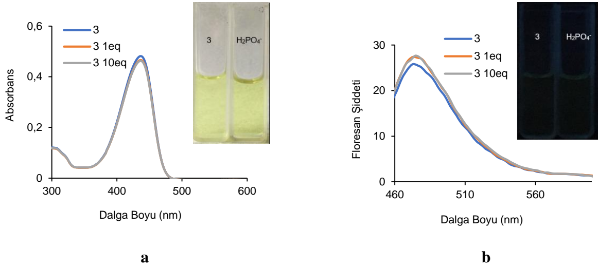
Şekil 5.52. 3 nolu bileşiğin TBAH 2 PO 4 ile titrasyonu sonucu elde edilen absorpsiyon ( 1 \times 10^{-5} M DMSO çözücüsünde) (a) ve emisyon ( 1 \times 10^{-6} M DMSO çözücüsünde, \lambda_{ex} = 440 nm) (b) spektrumları. (Grafiklerin içerisinde 3 nolu bileşiğin TBAH 2 PO 4 ile titrasyonu sonucu gözlenen fotofiziksel değişiklikler gün ışığında (a) ve UV ışığında (365 nm) (b) gözlenen fotoğrafları)
