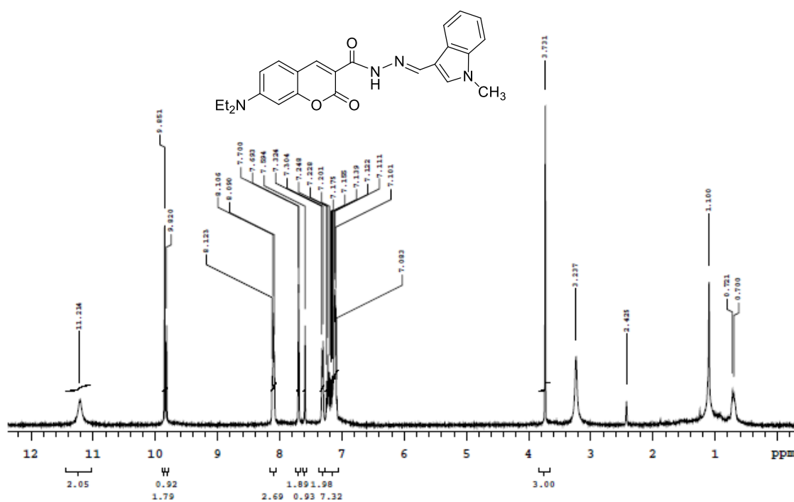
A15. 4 Nolu Bileşğin 1 H-NMR Spektrumu DMSO d 6 Çözücüsünde
