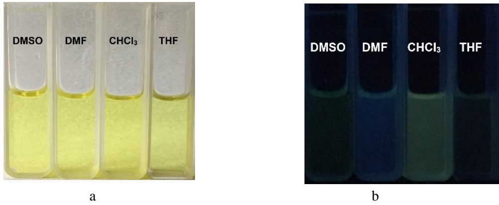
Şekil 5.24. 2 nolu bileşğin farklı çözücüler içerisindeki gün ışığında (a) ve UV ışığı (365 nm) altında (b) alınan fotoğrafları
