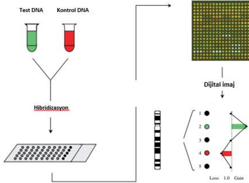
Şekil 2.7. a-CGH Prensipleri (Oostlander vd., 2004).
