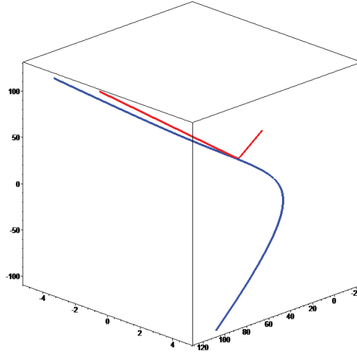
Şekil 5.4: Eğri ve \mathbf{t}_q \mathbf{b}_q -Smarandache eğrisi.
