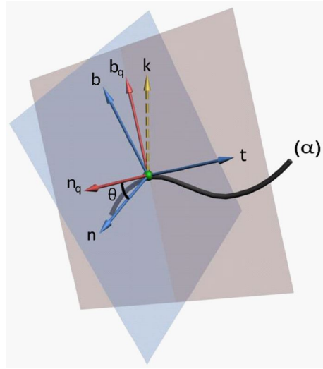
Şekil 3.4: q-çatısı ve Frenet çatısı
