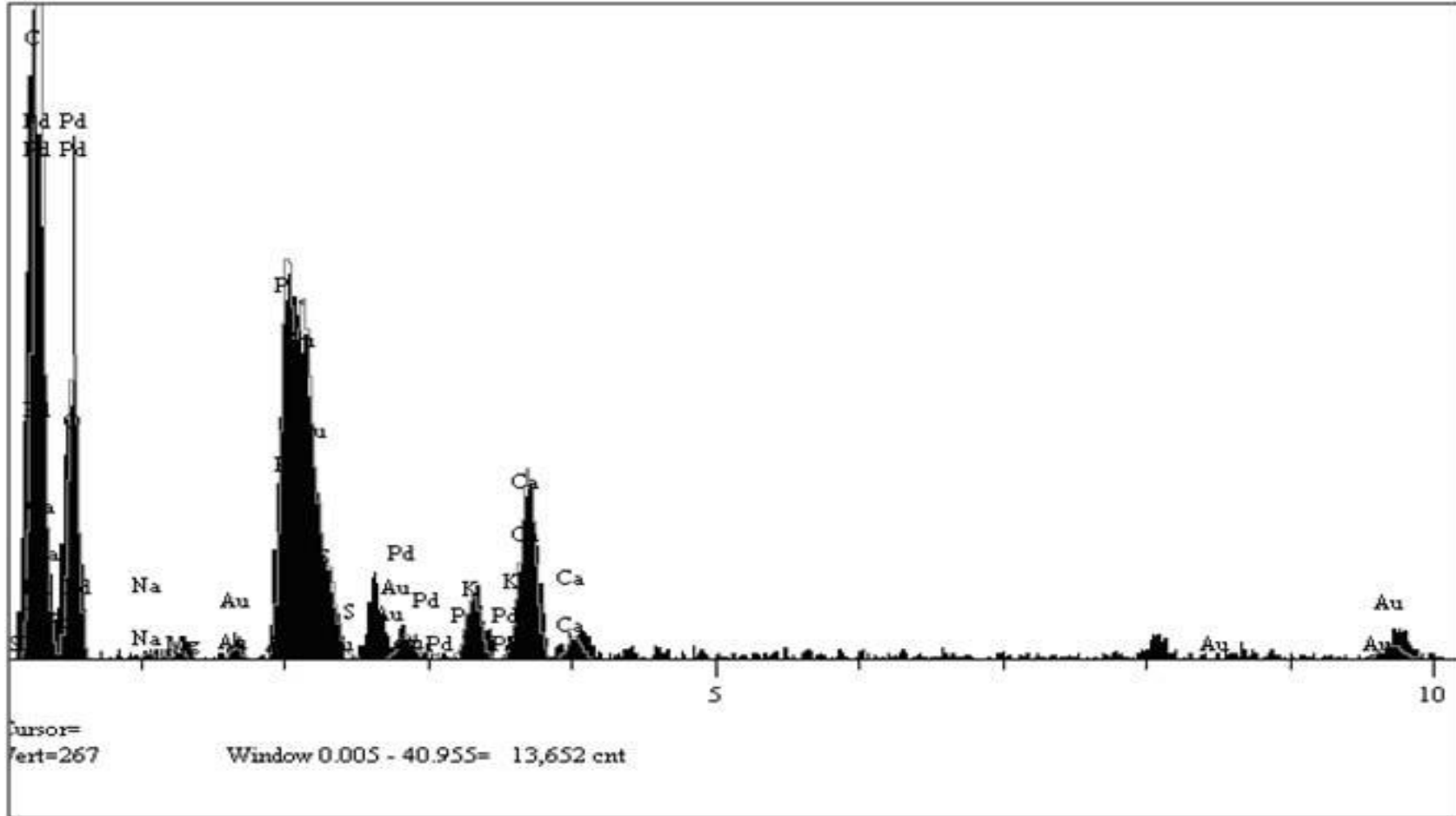
Şekil 6.30. Serbest N. sitophila 'nın EDX spektrumu
