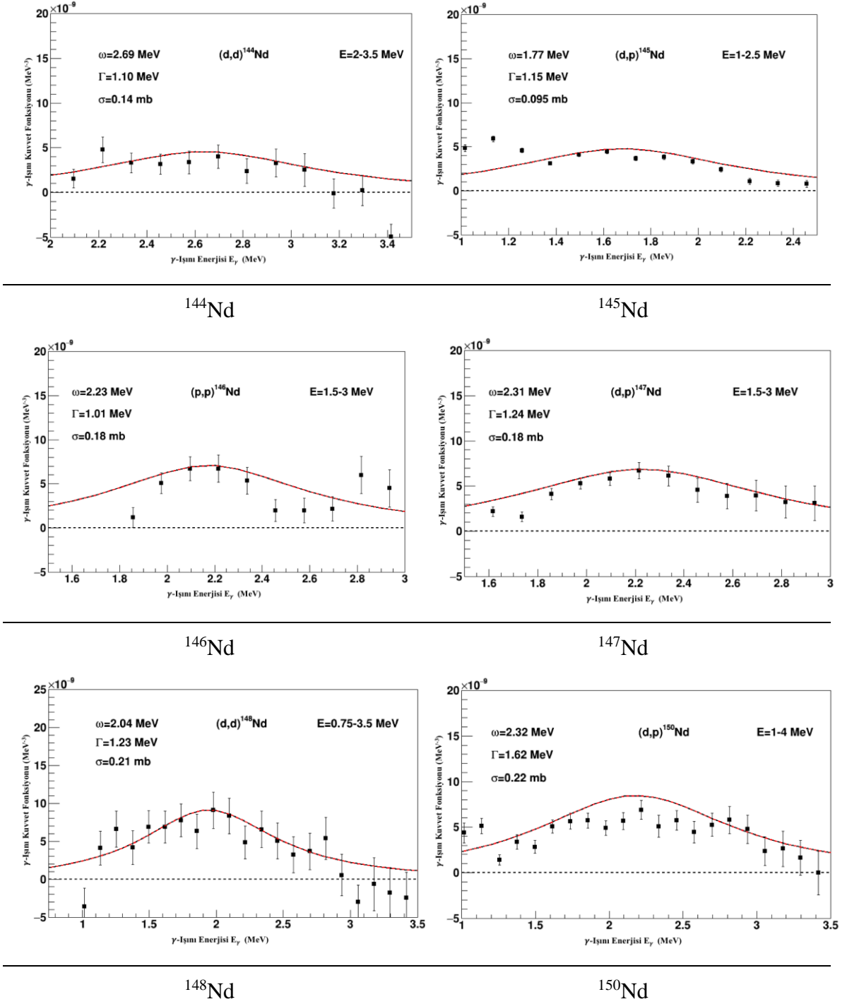
Şekil 6.9. 142,143,144,145,146,147,148,150 Nd çekirdeklerine ait makas rezonansı grafikleri.
