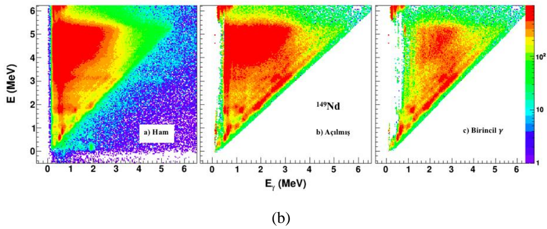
Şekil 5.3. (a) ^{149}\text{Nd} (b) ^{151}\text{Nd} izotoplarına ait ham, açılmış ve birincil gama matrisleri.
