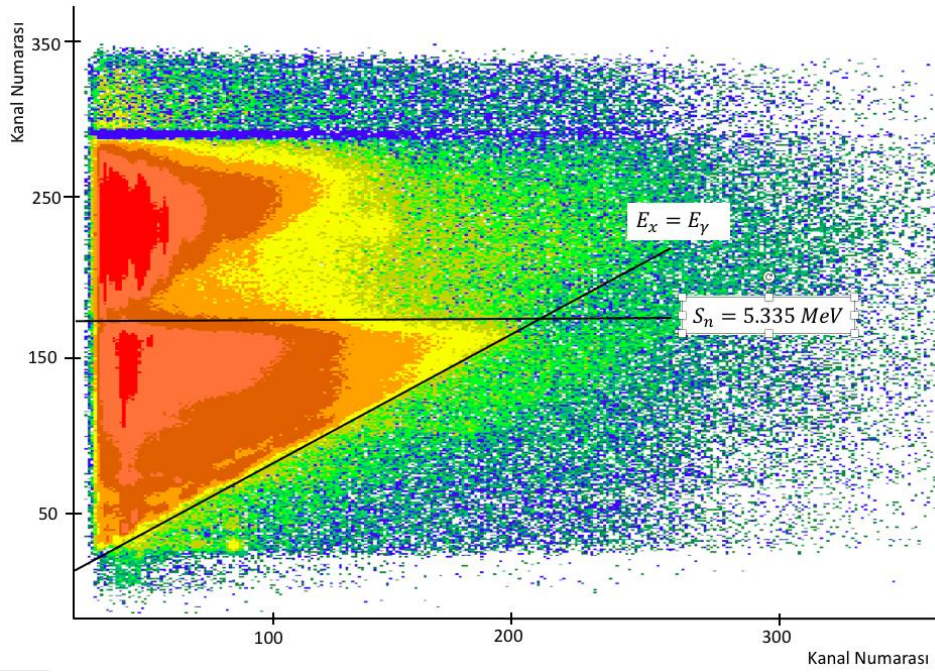
Şekil 4.10. ^{151}\text{Nd} izotopu için çakışma matrisi. Yatay çizgi nötron ayrılma enerjisini, diyagonal çizgi ise doğrudan taban duruma bozunmaları göstermektedir.
