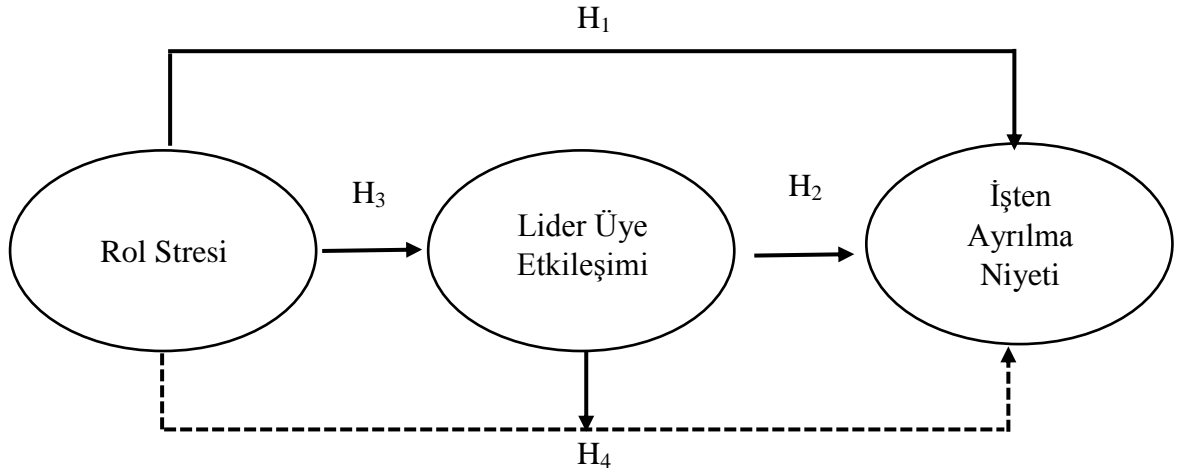
Şekil 6: Araştırmanın Modeli
